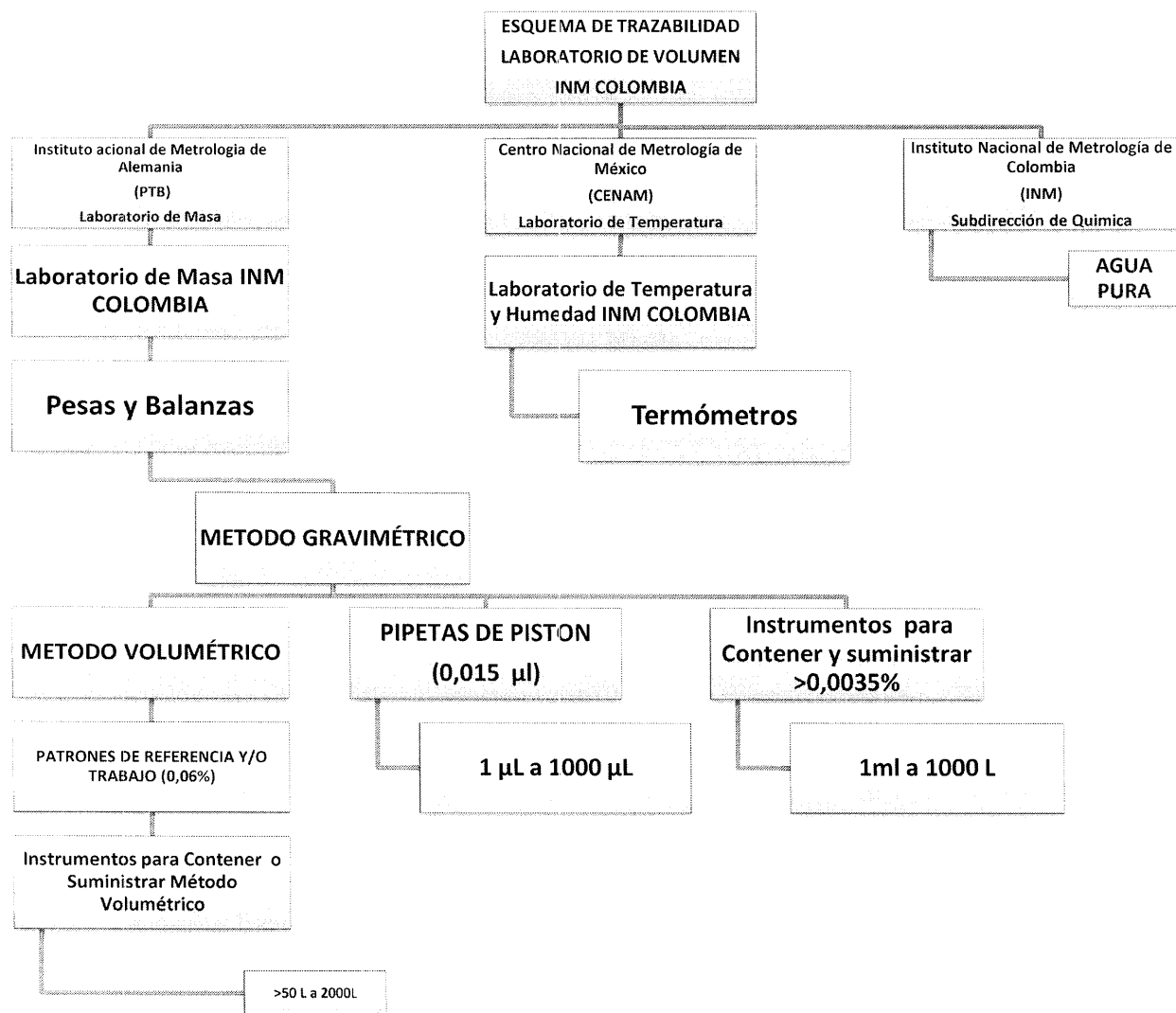
Figura 1: Descripción de la trazabilidad del Patrón Nacional de volumen del INM
